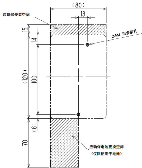
安装尺寸图（使用安装板）
