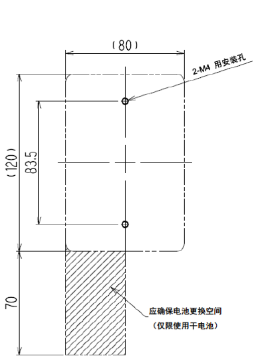
安装尺寸图（未使用安装板） 适合 JIS 1 个用开关盒
